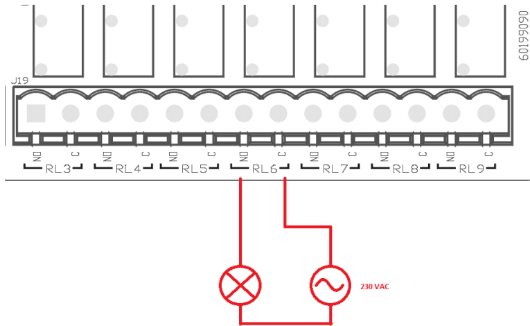
Obrázek 6: Příklad připojení O1 s napětím 230V
