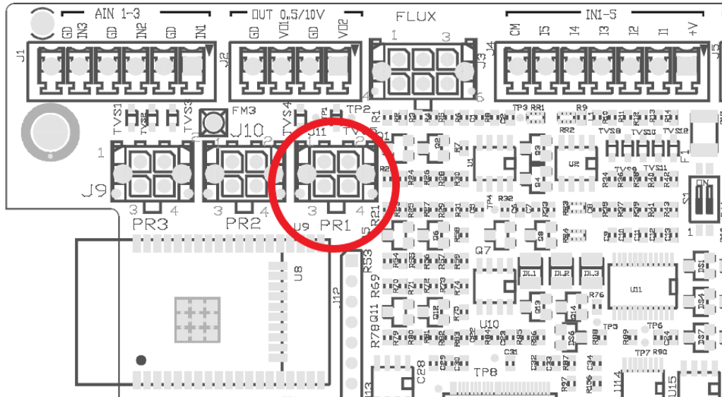
Figura 8: Ligação sensor de pressão
