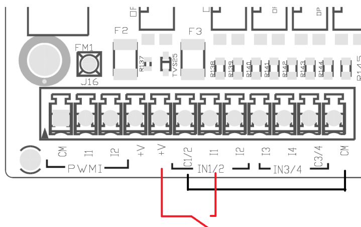
Rysunek 4: Przykład połączenia czystego styku
