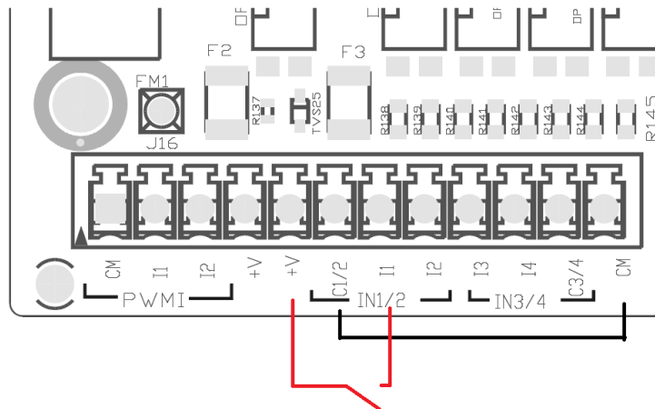
Figura 4: Ejemplo de conexión de contacto limpio
