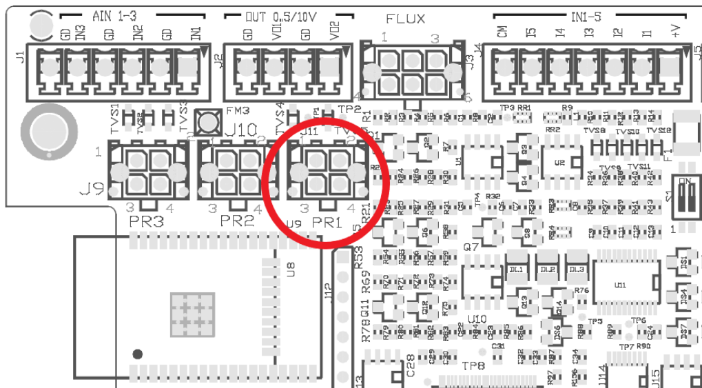
Figura 8: Conectare senzor de presiune
