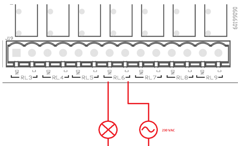
Фигура 6: Пример свързване O1 при натоварване 230V
