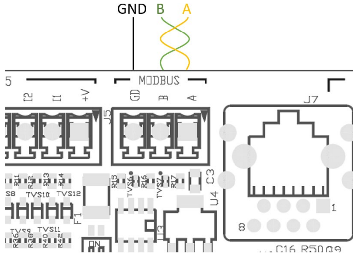
Figura 10: Cableado Rs485 Modbus
