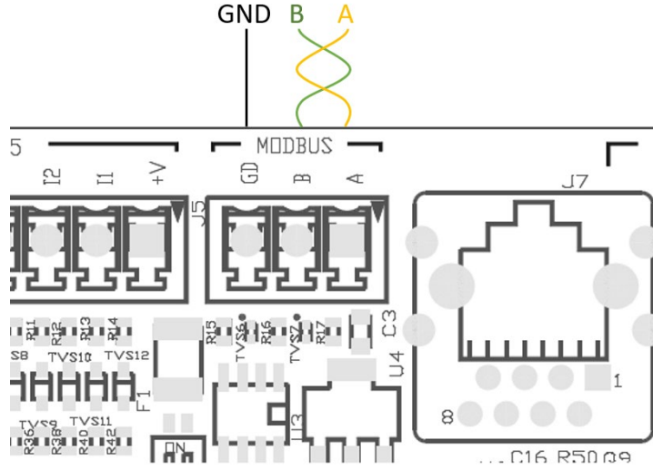
Şekil 10: Rs485 Modbus kablajı
