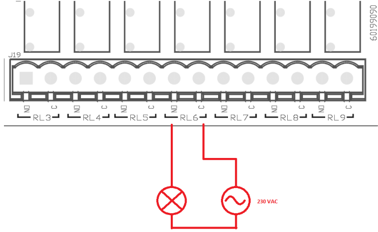
Şekil 6: 230V yük ile O1 bağlantı örneği
