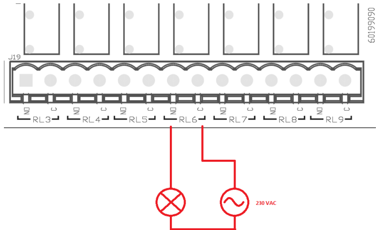
Figura 6: Esempio connessione O1 con carico a 230V
