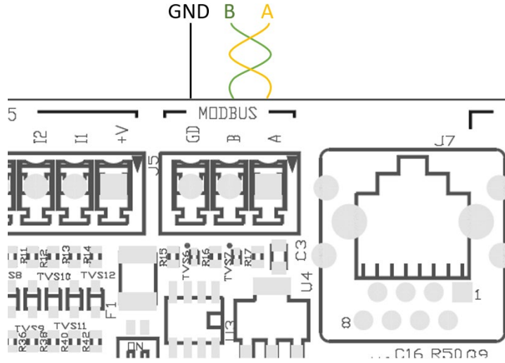
الشكل 10: أسلاك Rs485 Modbus
