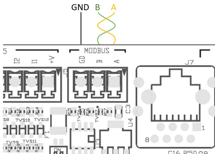
Rysunek 10: Okablowanie Rs485 Modbus
