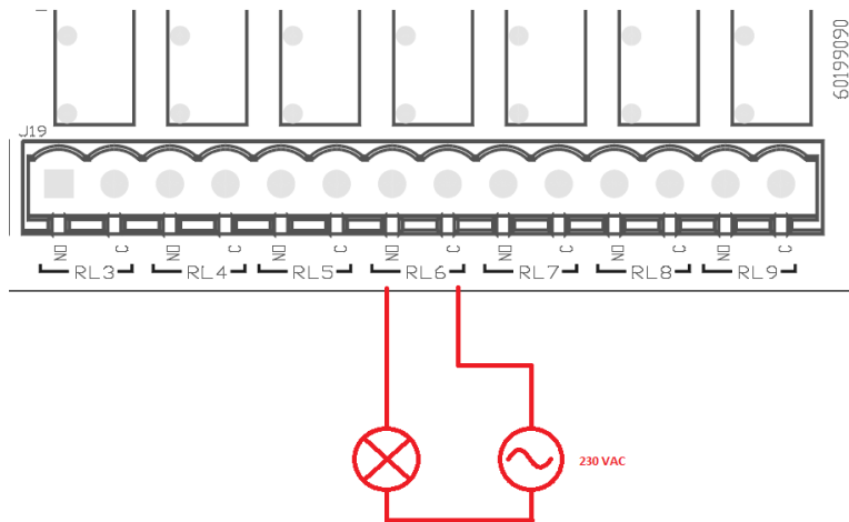
6. ábra: 01 kimeneten, 230 V terheléssel elvégzett csatlakozási példa
