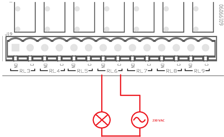
Εικόνα 6: Παράδειγμα σύνδεσης O1 με φορτίο στα 230V
