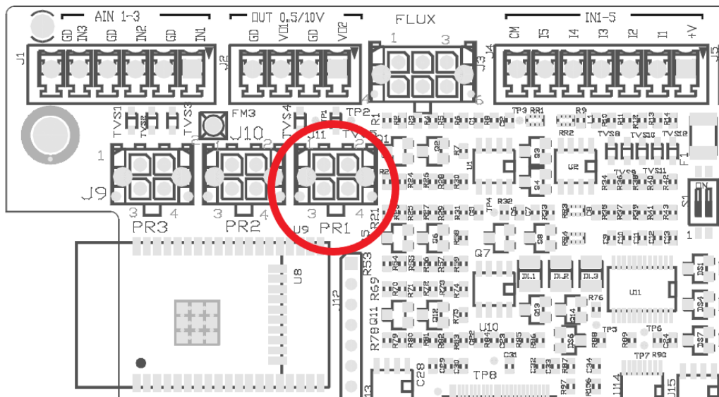
Obrázek 8: Připojení dálkově ovládaného tlakového snímače
