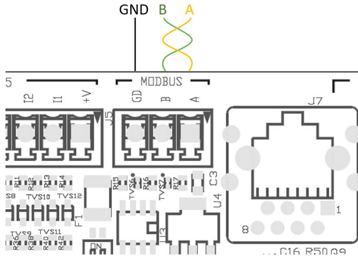
Obrázek 10: Kabely Rs485 Modbus
