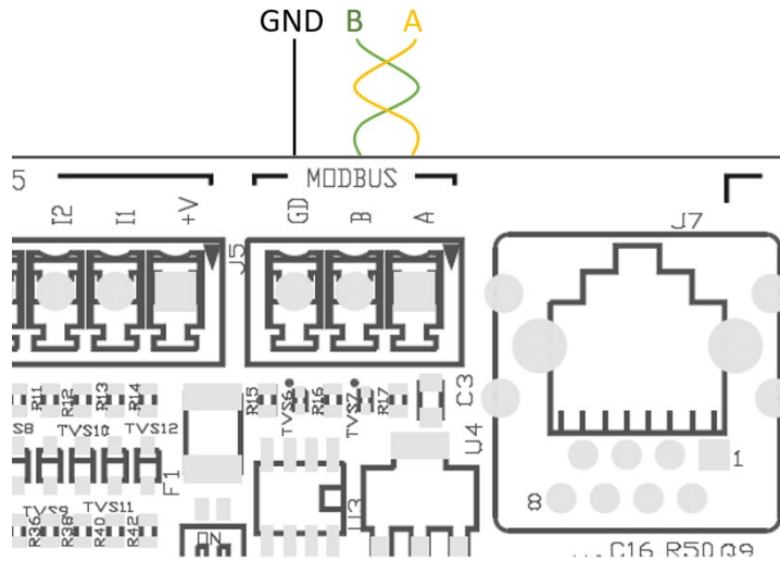
Figura 10: Cablare Rs485 Modbus
