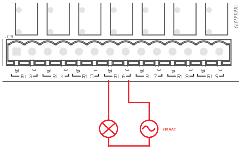
Figura 6: Exemplo de conexão O1 com carga a 230V
