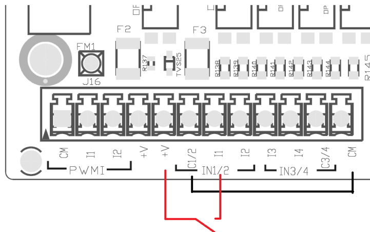
Fig. 4: Exempel på anslutning med potentialfri kontakt
