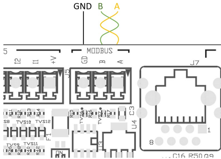
Figura 10: Cablaggio Rs485 Modbus
