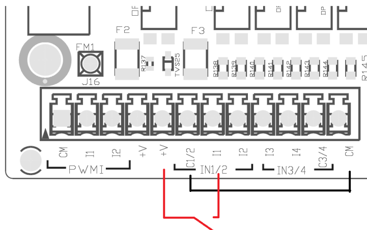
Figura 4: Exemplo ligação contacto livre
