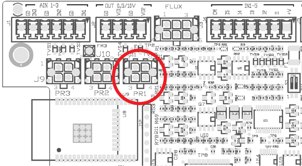
Фигура 8: Свързване на сензора за налягането
