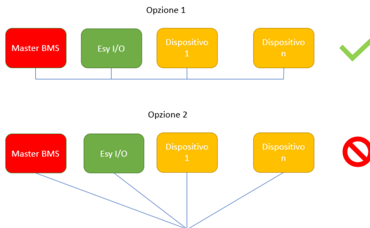
Рисунок 11: Примеры подключения проводов bus
