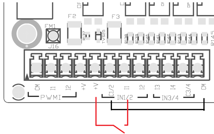
الشكل 4: مثال لتوصيل اتصال نظيف
