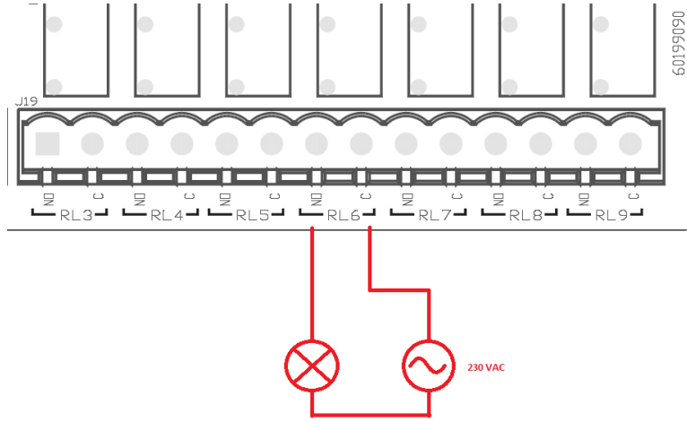
الشكل 6: مثال اتصال O1 بشحن 230 فولت
