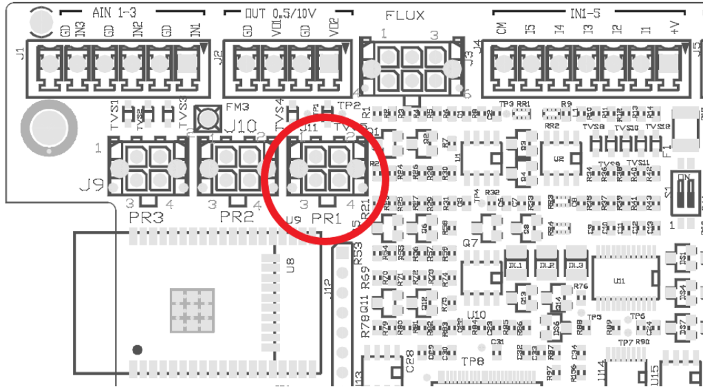
Fig. 8: Anslutning av trycksensor
