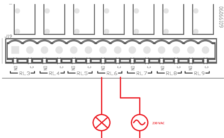
Kuva 6: esimerkki liitännästä O1 230 V:n kuormalla
