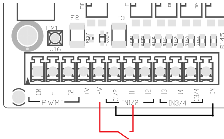
Фигура 4: Пример за свързване сух контакт
