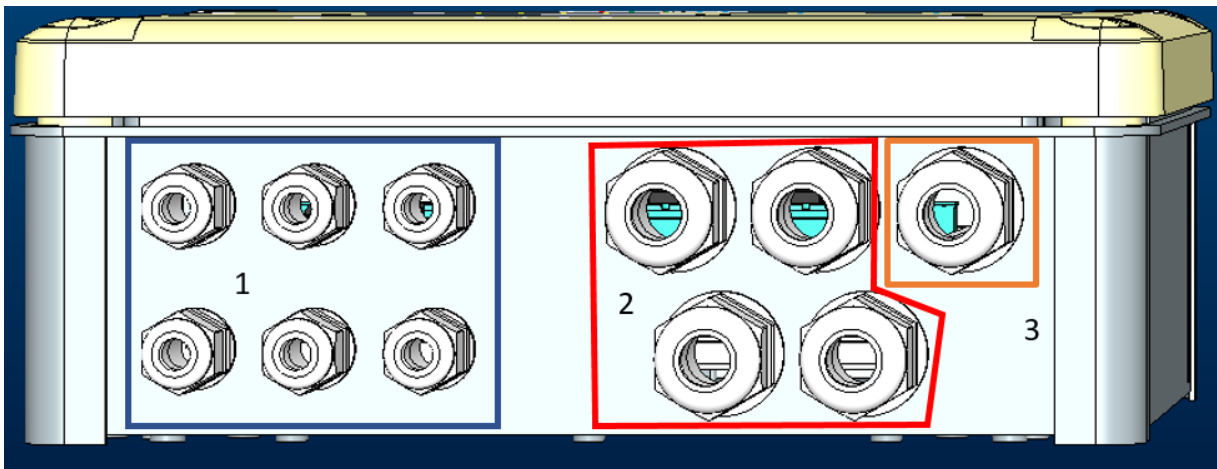
Kuva 1: holkkitiivistelevy
