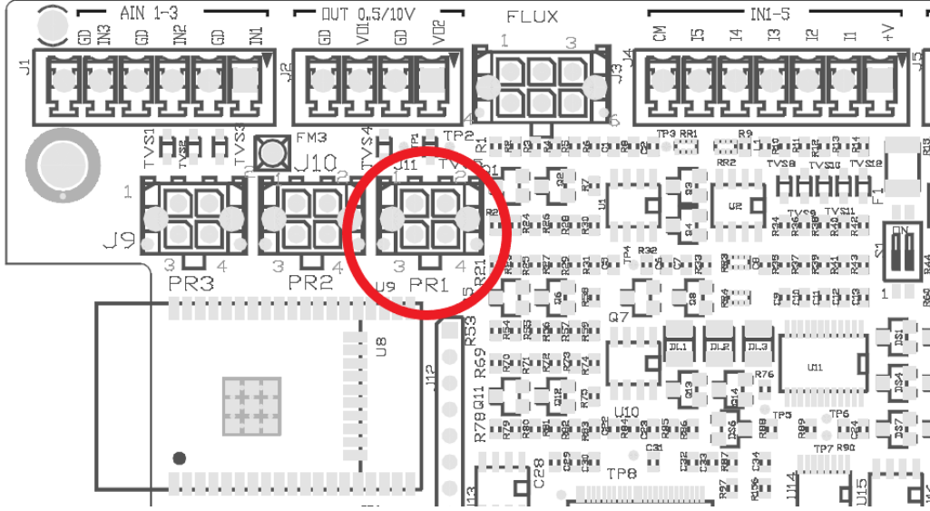
Şekil 8: Basınç sensörü bağlantısı
