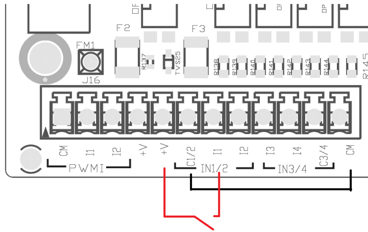
Şekil 4: Temiz kontak bağlama örneği
