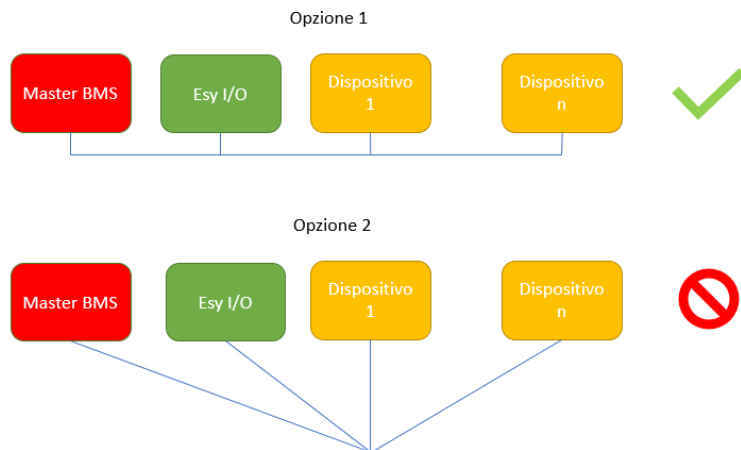
Abbildung 11: Beispiele Bus-Verkabelung
