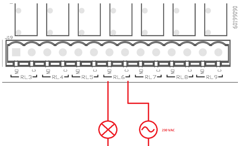
Figura 6: Exemplu de conexiune O1 cu sarcină 230V
