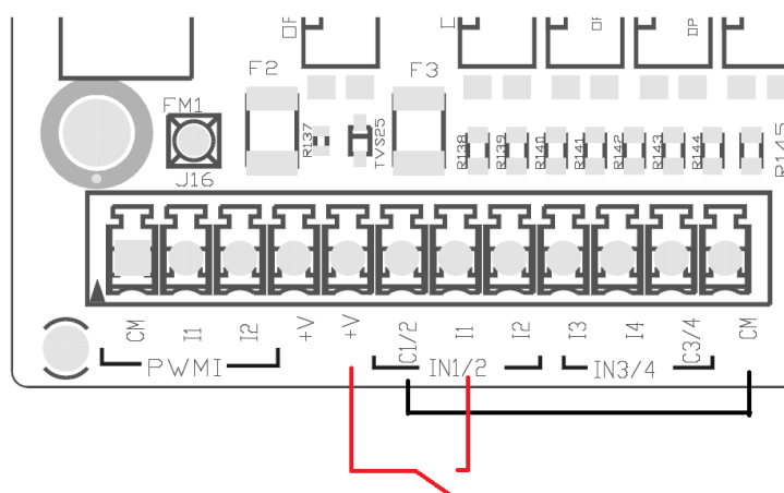
Εικόνα 4: Παράδειγμα σύνδεσης ψυχρής επαφής
