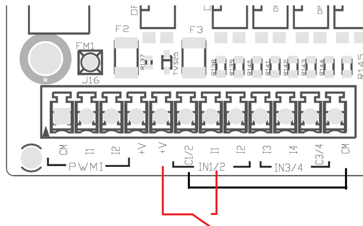
Figura 4: Exemplu de conexiune de contact curat
