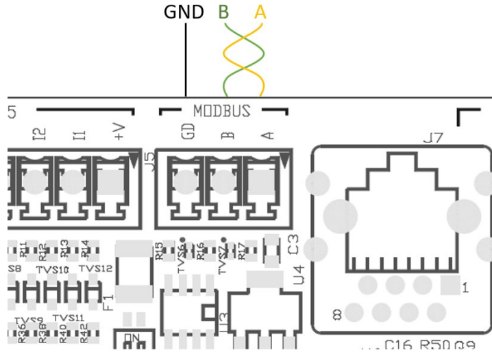
Εικόνα 10: Καλωδίωση Rs485 Modbus
