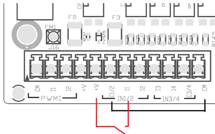
Kuva 4: esimerkki jännitteettömän koskettimen liitännästä
