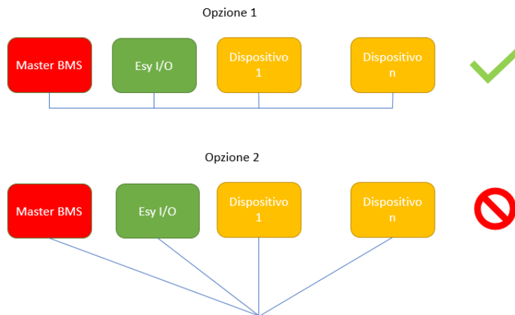
Фигура 11: Примери за окабеляване на шината
