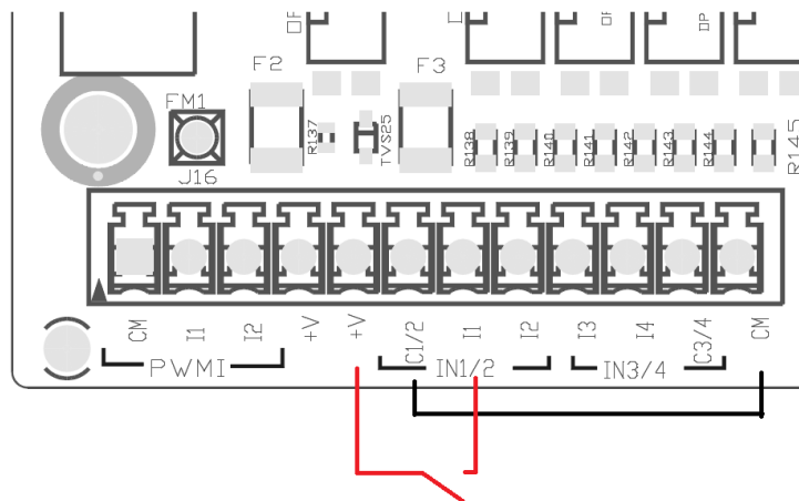
Obrázek 4: Příklad připojení kontaktu bez napětí
