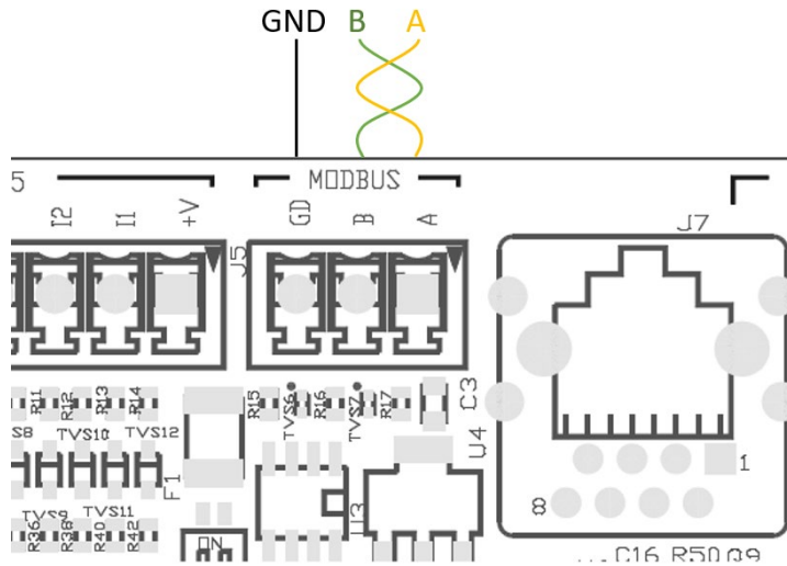
10. ábra: Rs485 Modbus kábelezés
